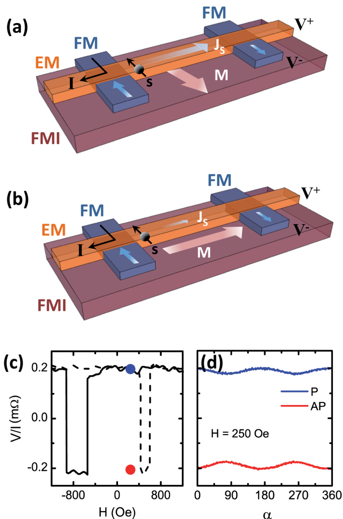
5. irudia. (a)-(b) Spinak manipulatzeko erabilitako gailuaren eskema, zeina alboko spin-balbulak bat material ferromagnetiko isolatzaile (FMI) baten gainean fabrikatzean datzan. (a) FMlaren magnetizazioa ( M ) eta spinen polarizazioa ( s ) paraleloak direnean, ez dago spin-xurgapenik. (b) M eta s perpendikularrak direnean, ordea, FMlako spinak xurgatu egiten ditu, eta neurtzen dugun spin-seinalea txikitzen da. (c) Mota horretako gailu batean neurturiko seinalea kanpoko eremu magnetiko baten arabera. (d) Kanpoko eremu magnetikoa 250 Oe-tan finkatuz baina haren norabidea \alpha angeluaz aldatuz neurturiko seinalea, elektrodo FMen magnetizazio paralelo (lerro urdina) zein antiparalelorako (lerro gorria). % 8ko modulazio nabarmen bat atzematzen da.
