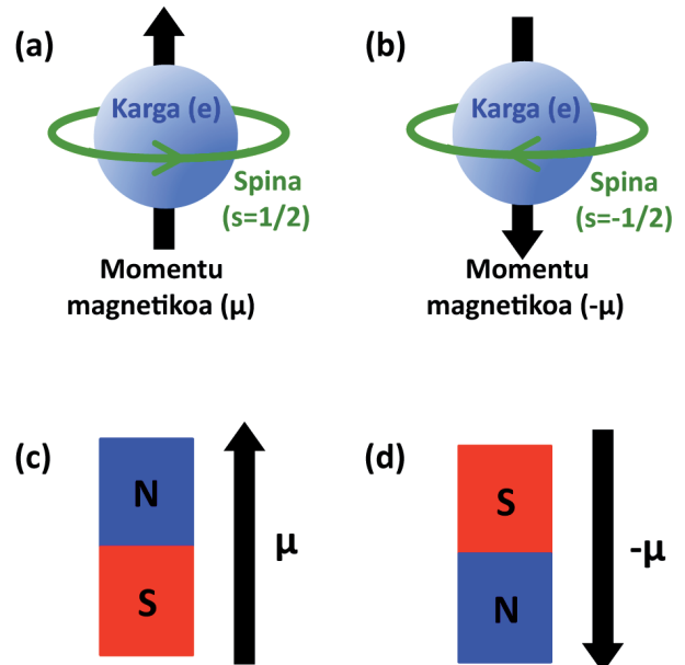
1. irudia. (a) Goranzko eta (b) beheranzko spinak ( s = 1/2 eta s = -1/2 ) dituen elektroien bat, (c) eta (d) elektroien horren momentu magnetikoa ( \mu eta -\mu ).
